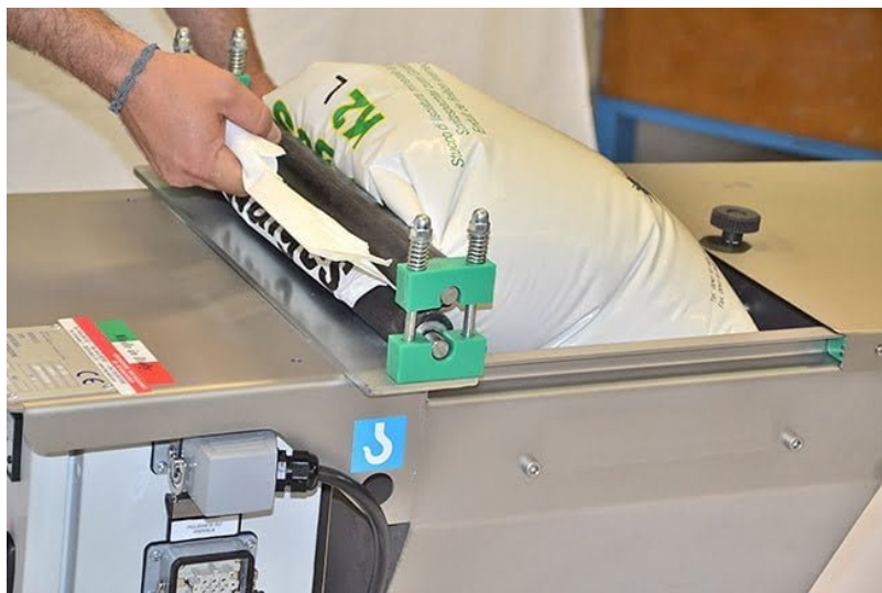
066252 – strizzasacchi MTV 500
